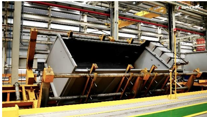
溶接用反転治具(ダンプボデー)
