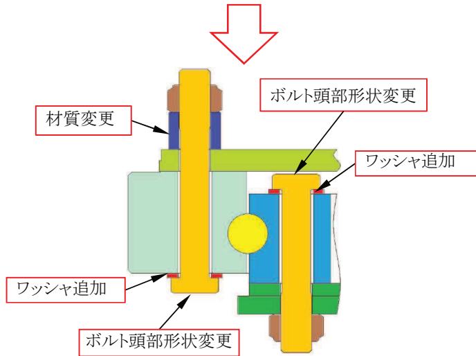
対策形状締結部詳細
