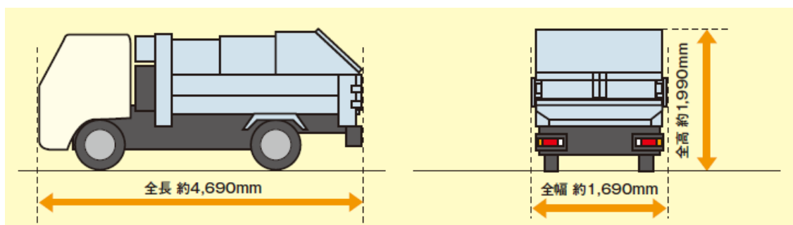
車両サイズ
