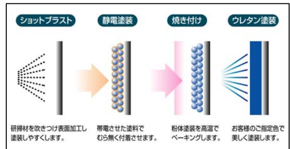
粉体塗装のフロー
